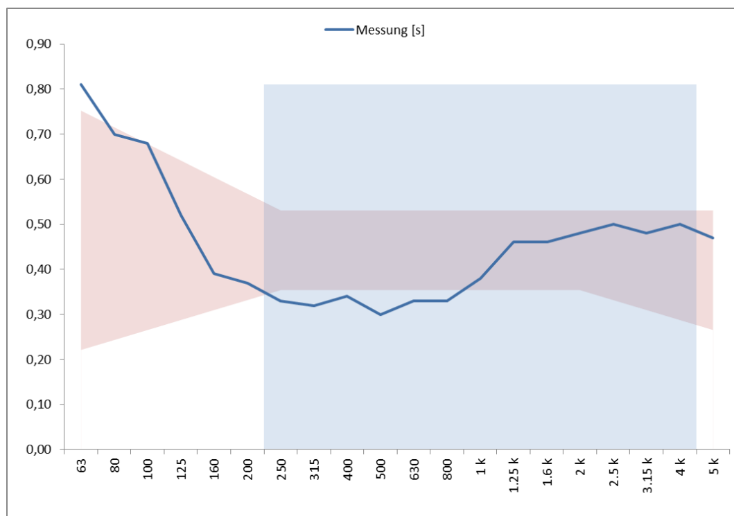
Abbildung 2: Nachhaltzeiten Klasse 2 TFO
