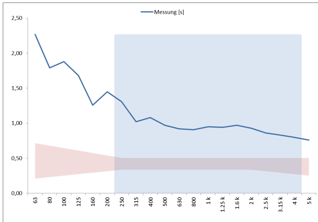
Abbildung 1: Nachhaltzeiten Klasse 3B RG
